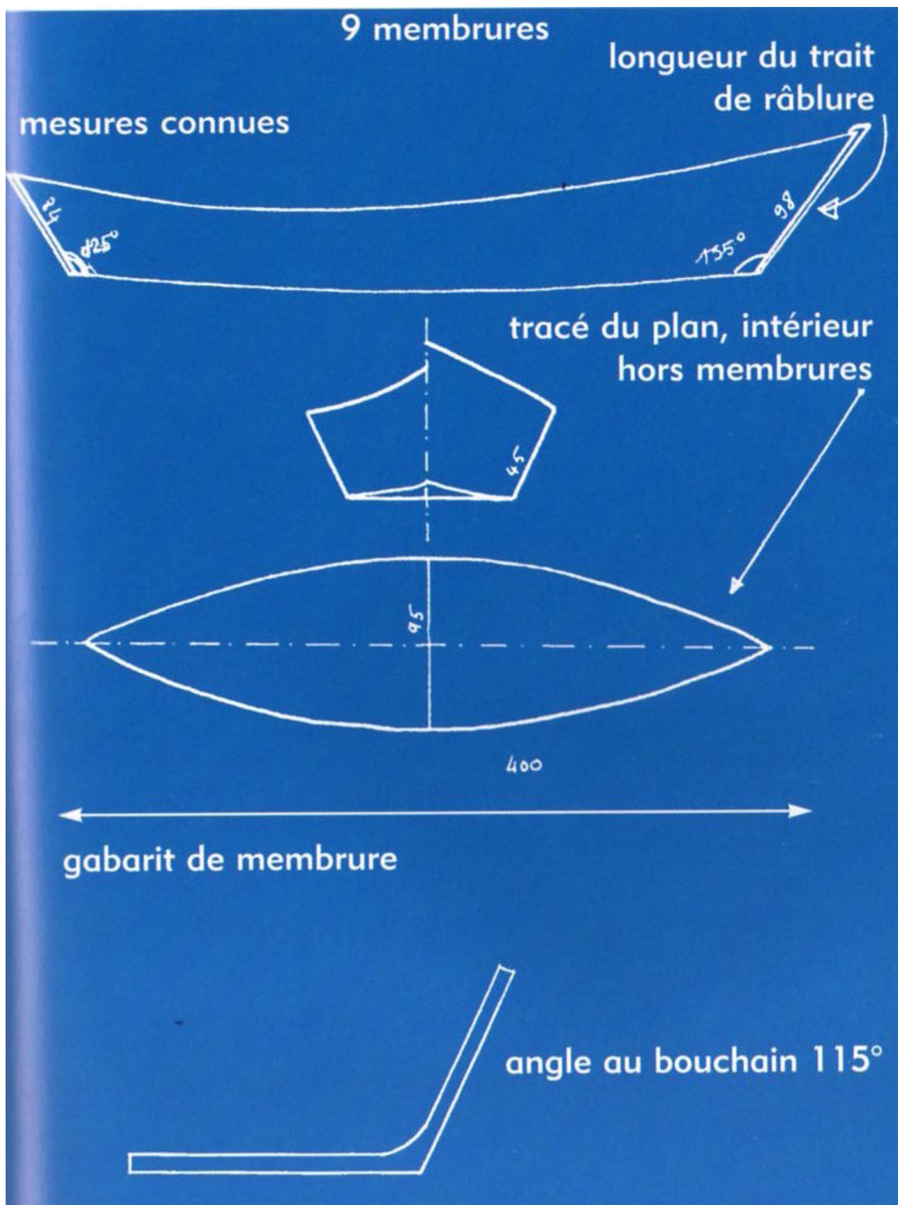
Plan de Monsieur Aversa
